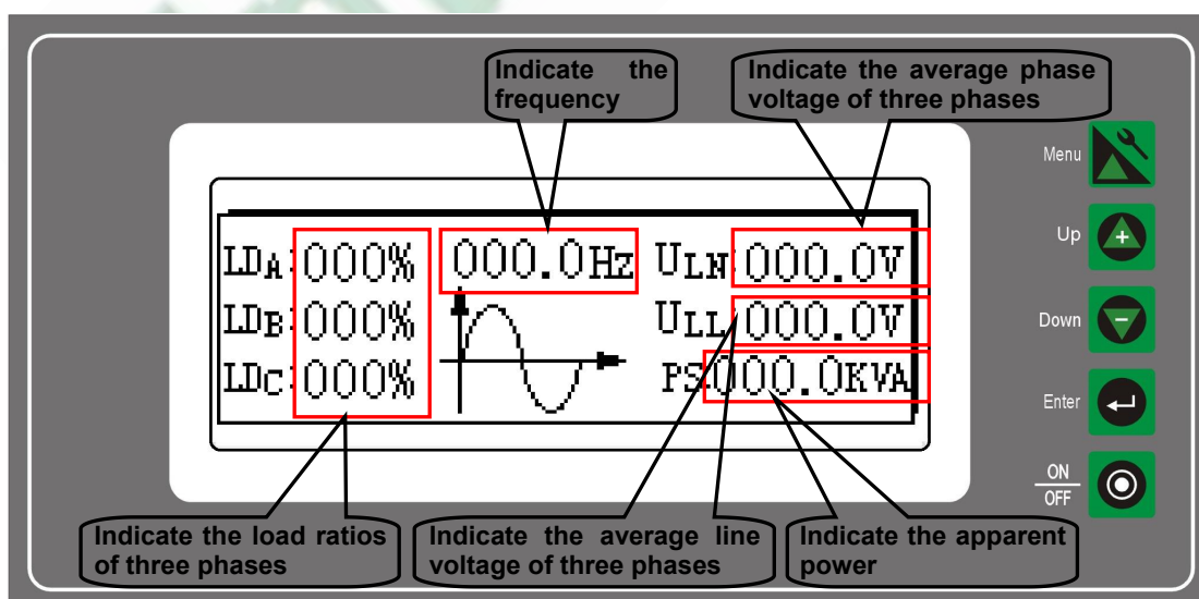
Fig. 5 Interface 2
